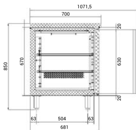
▲ boční pohled
